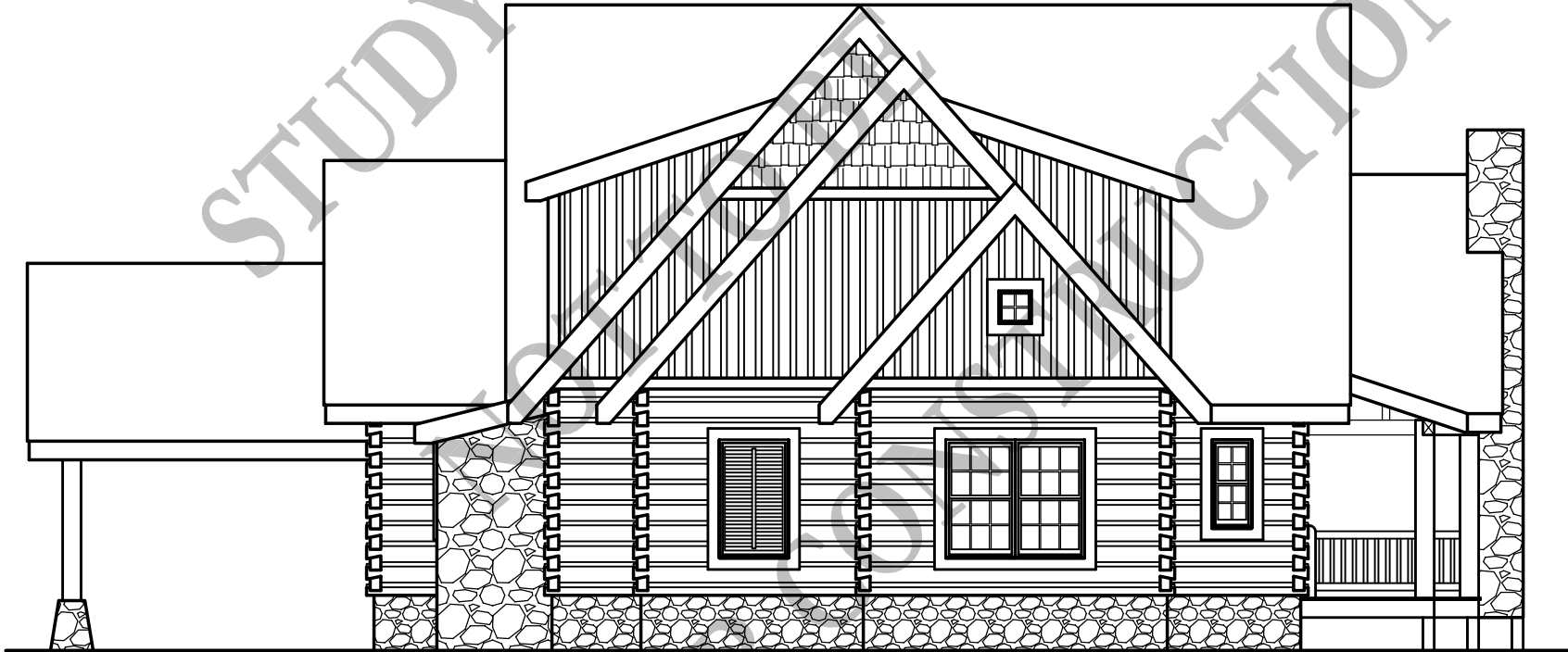
RIGHT ELEVATION
