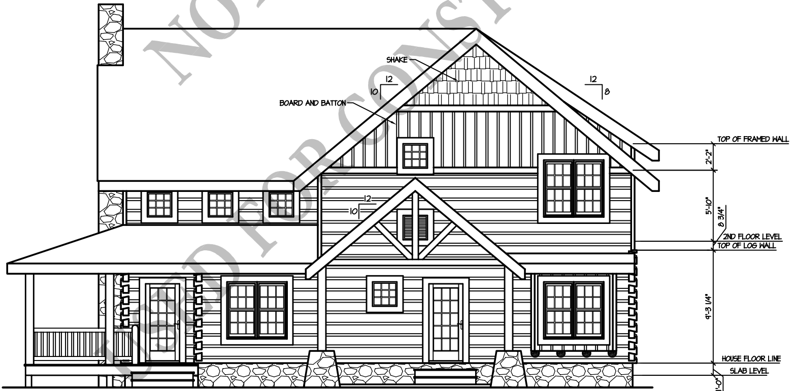
RIGHT ELEVATION
