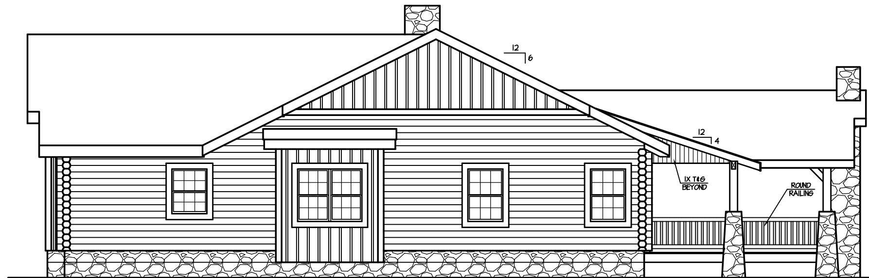
RIGHT ELEVATION
