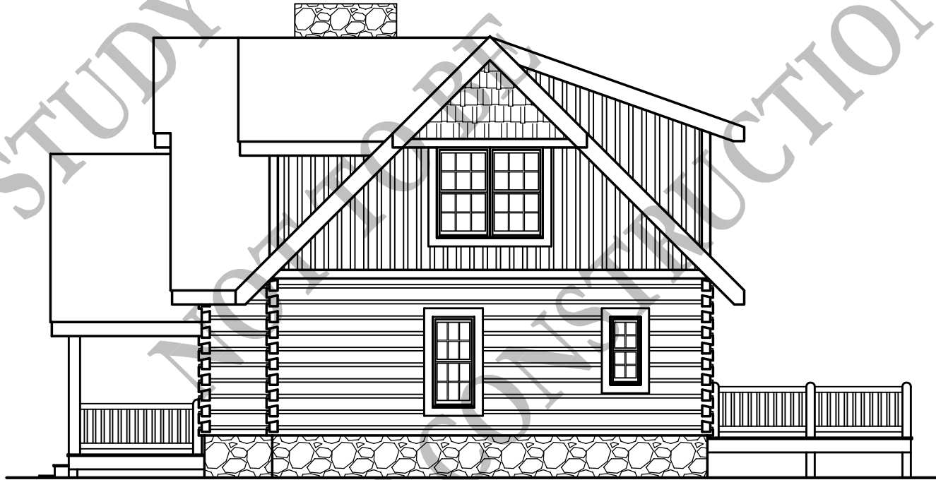
RIGHT ELEVATION
