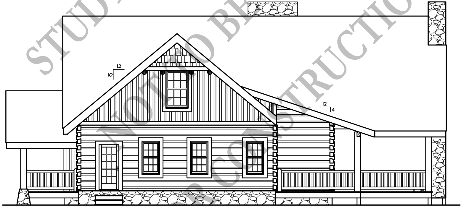
RIGHT ELEVATION
