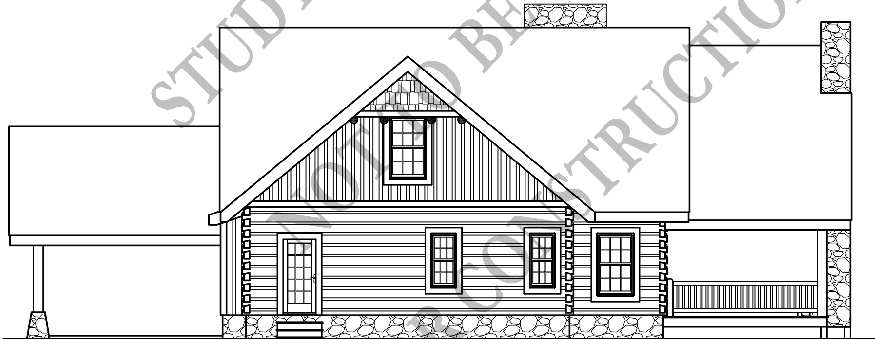
RIGHT ELEVATION
