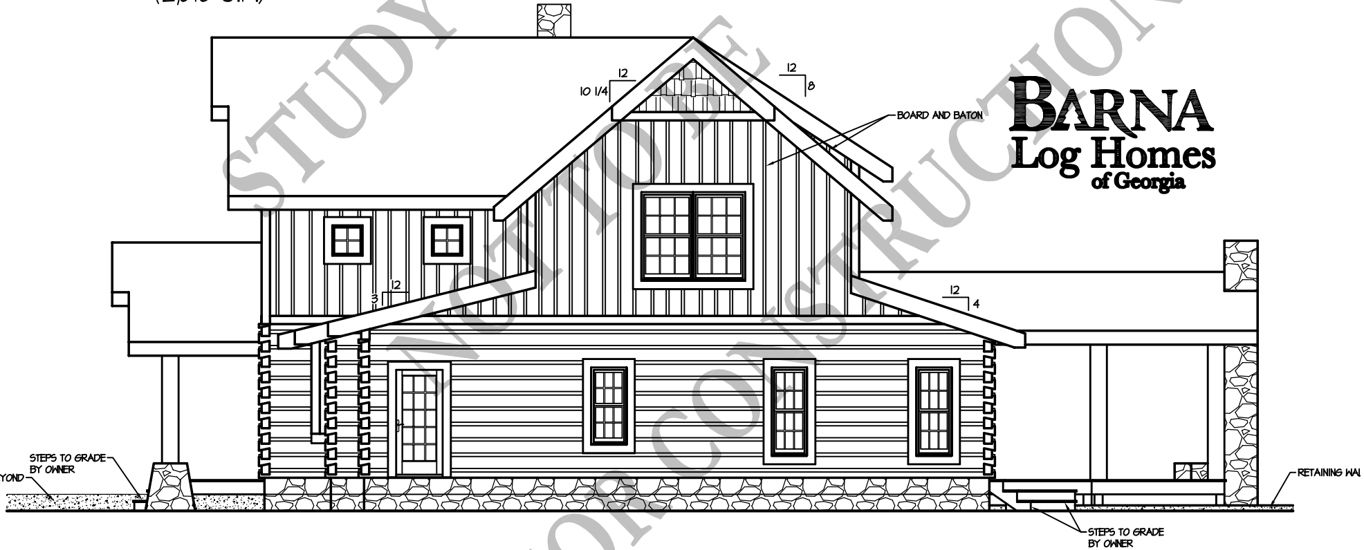
RIGHT ELEVATION
