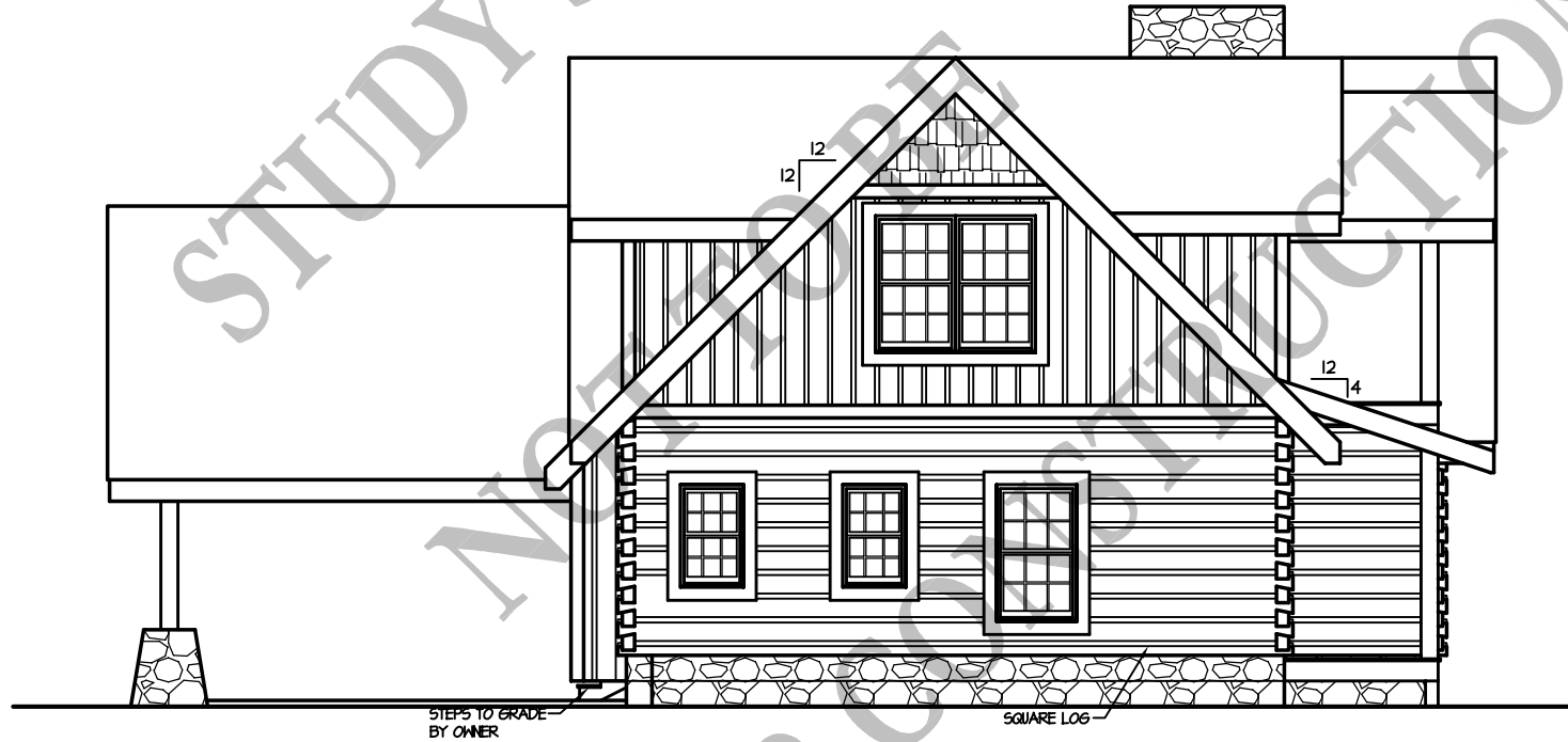
RIGHT ELEVATION
