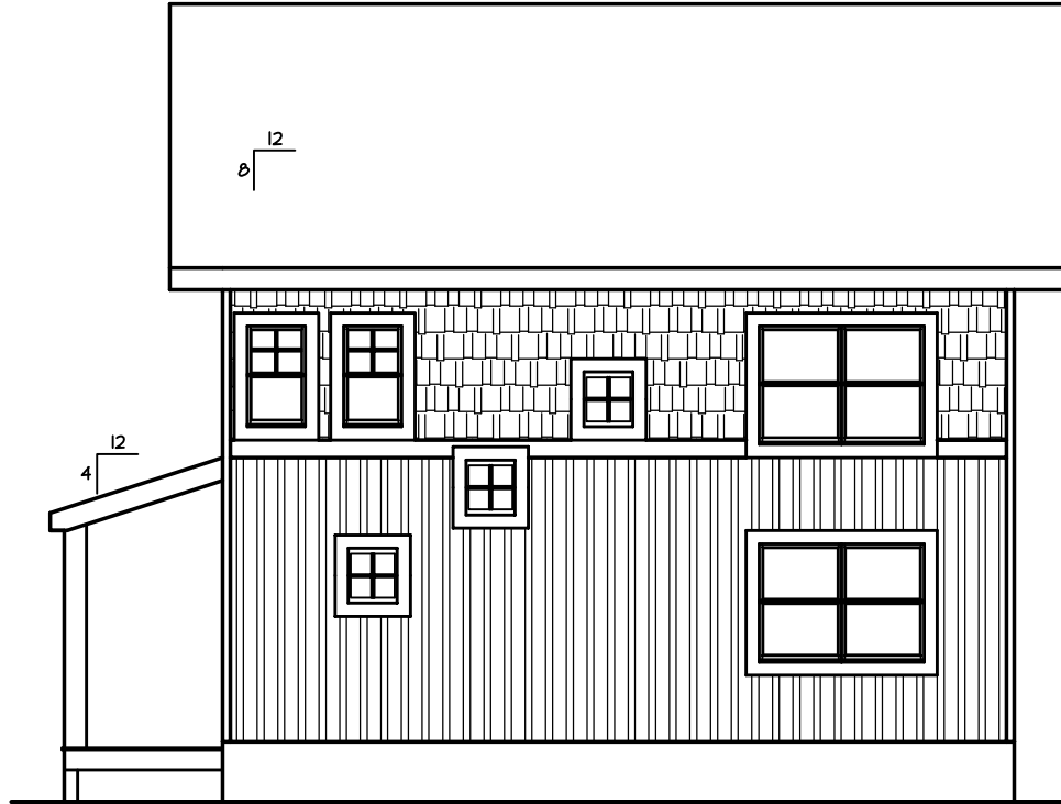
RIGHT ELEVATION
